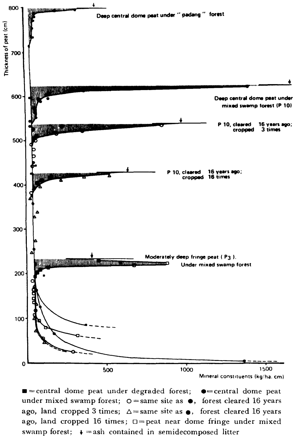
図5 西カリマンタンのドーム状泥炭中の無機成分の分布 (Driessen [1978] より引用)
