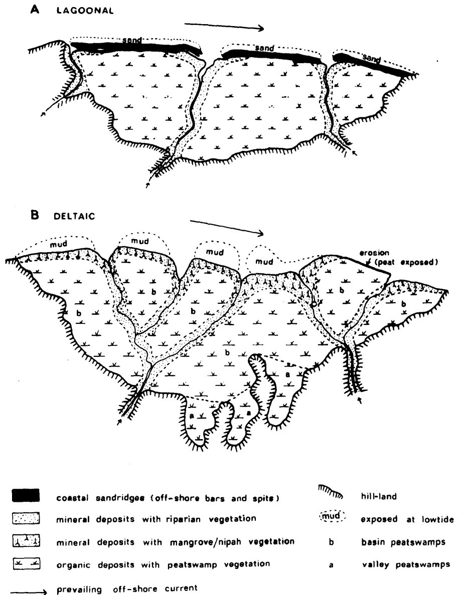
図3 泥炭湿地の地形環境 (Andriess [1974] より引用)
