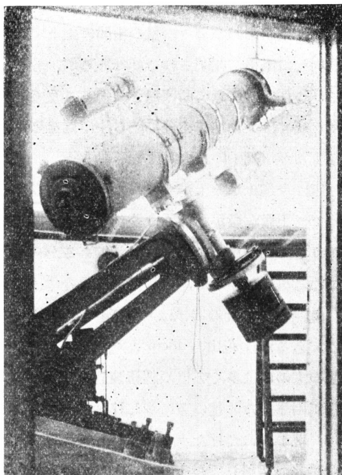
黒いカメラは10cm人像玉、白いカメラは6cm ツアイス、ベツバル、ピラーを這つてゐる紐は 赤經微動のエンドレス・コード
