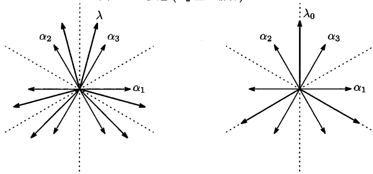
図 2: W -軌道 ( A_2 型の場合)
