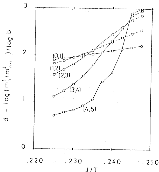
第3図 ブロックスピン磁化の比のくりこみのふるまい [7]。ランダム磁場は \pm h_R 分布で h_R/J=0.8 。図中のかっこ内の数字はブロックスピン変換の次数を表す。
