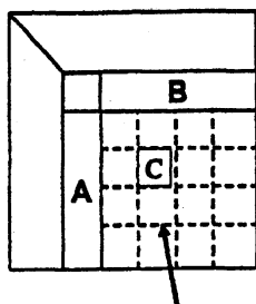
図5. ブロックLU分解法の適用イメージ
