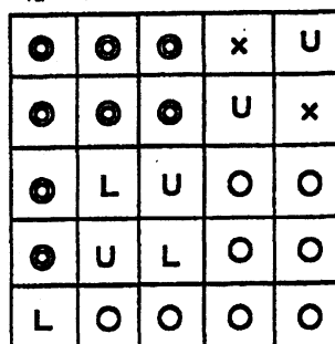
図4. n=5 のときのCの計算式の配置
