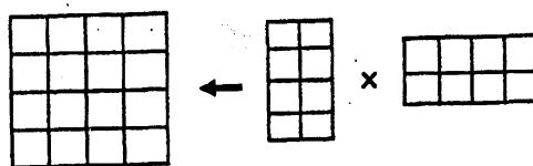
図2 拡張ストラッセン法のイメージ
