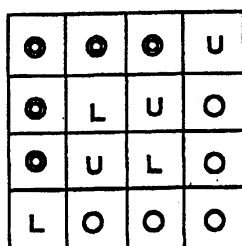
図3. n=4 のときのCの計算式の配置
