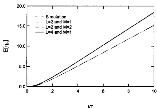
図3 履歴消費エネルギーの平均値 ( r=0.5 )
