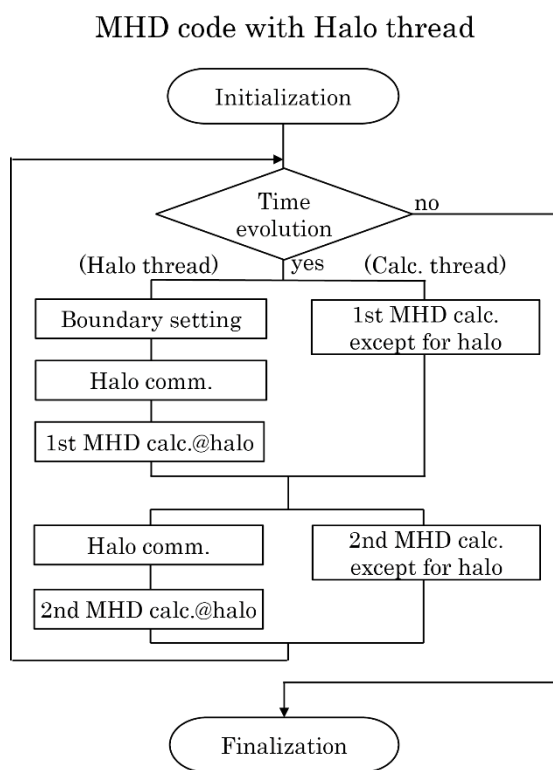
図 1 Halo Thread を導入した MHD 計算フローチャート Figure 1 Flowchart of MHD code with Halo thread.
