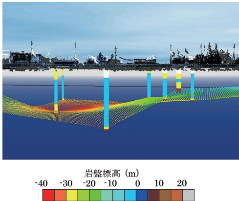
図11 MMSによる地表データと地下構造の統合データモデルの一例
