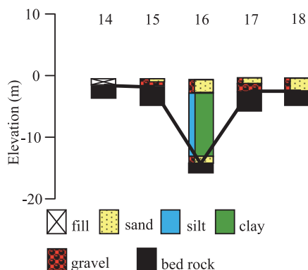
図 6 測線 C に沿ったボーリングによる断面表示
