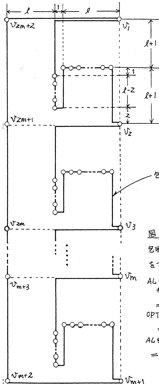
図 16. N.Christofides の方法による最悪の振舞をする例
