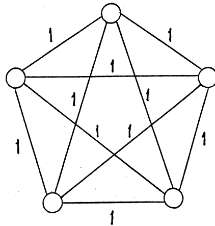
図2. 平面格子上で扱えない一般グラフの例
