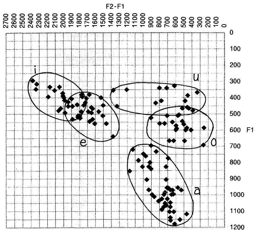
Tutuba vowel chart
