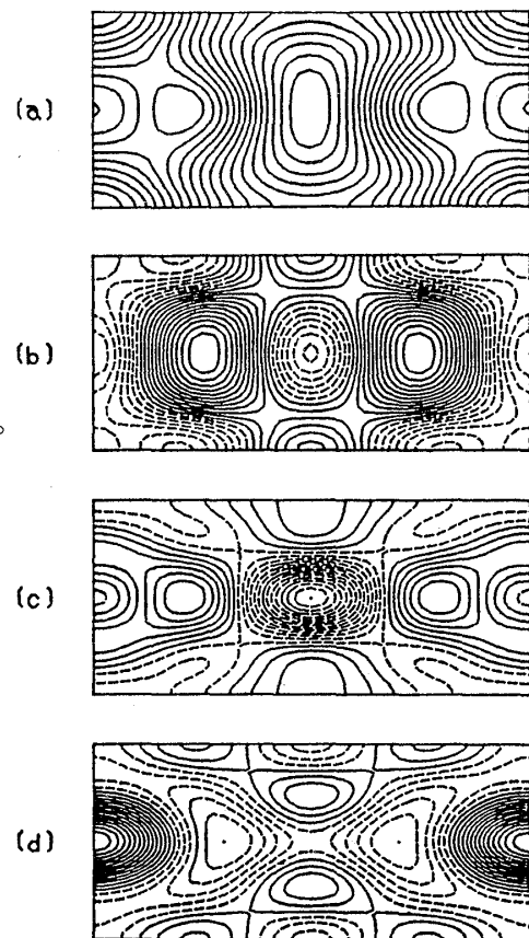
図2 温度場 \theta(x, y, z = 0.25) の等値線。ただし -\Gamma_X/2 < x < \Gamma_X/2 , -\Gamma_Y/2 < y < \Gamma_Y/2 , 1/2 < z < 1/2 。 \Gamma_X = 1.2 , \Gamma_Y = 2.7 , \sigma = 0.5 , s = R/R_0 = 4.529 の場合で、実線は正、破線は負の値を示す。
