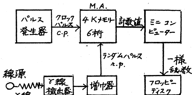
図1. 乱数発生装置の原理図
