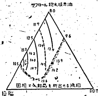
第七圖 サフロール+赤水拔赤油樟腦 DDT三成分系の完全液相に対するBHCの溶解度30°
