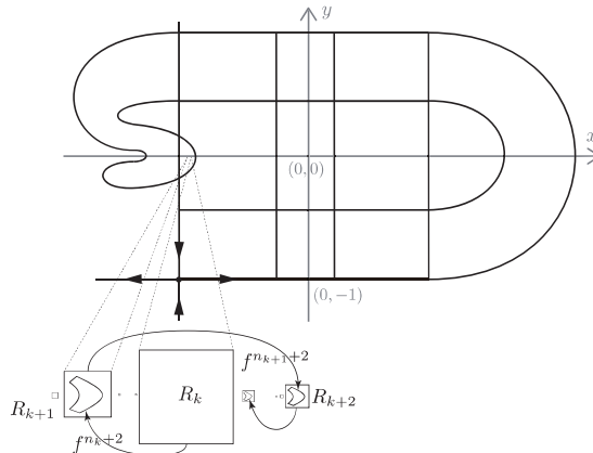
図 1 Colli-Vargas 微分同相写像
