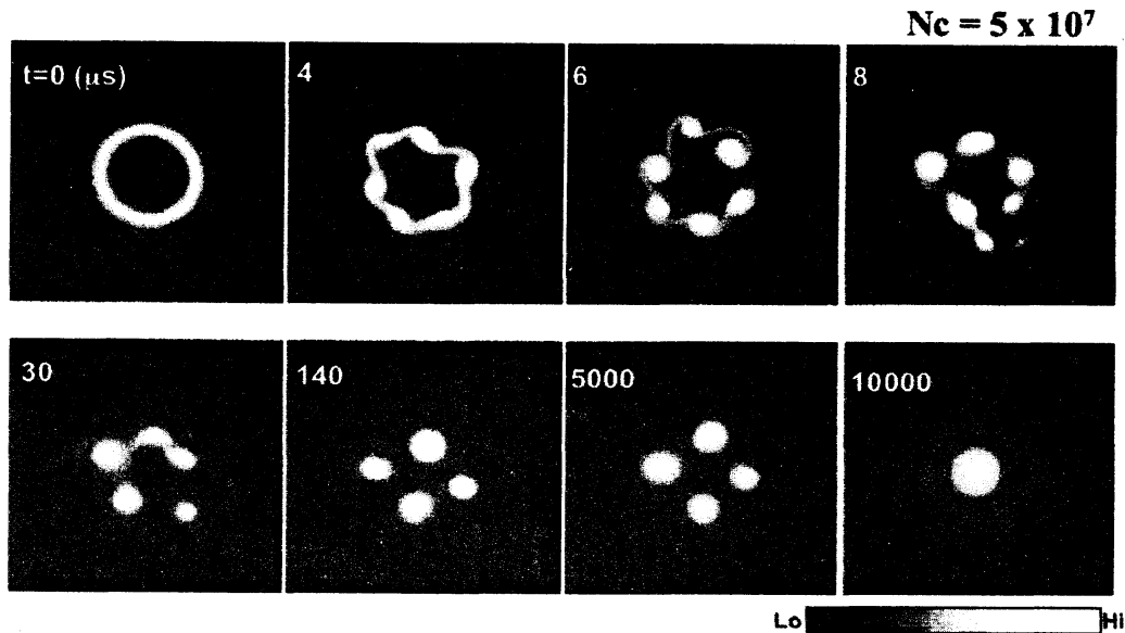
図 1: Hollow 状の渦度分布からの渦結晶形成
