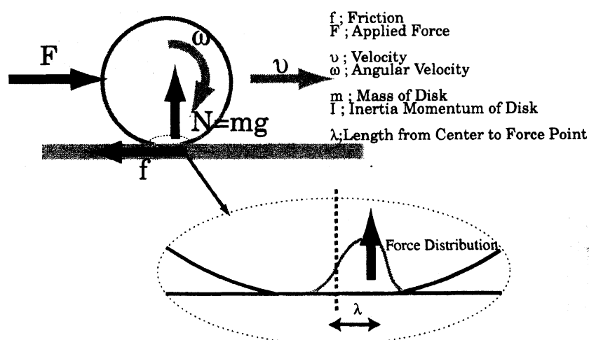
図 1: 転がりにおける釣合
