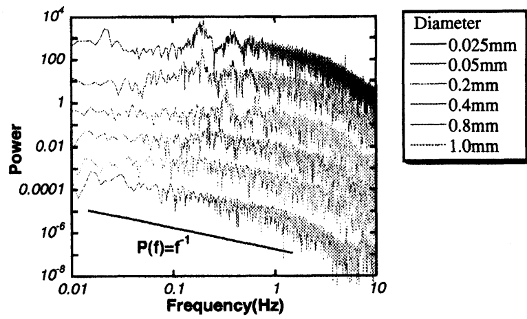
図 6: 周波数 Spectrum の粒径による違い
