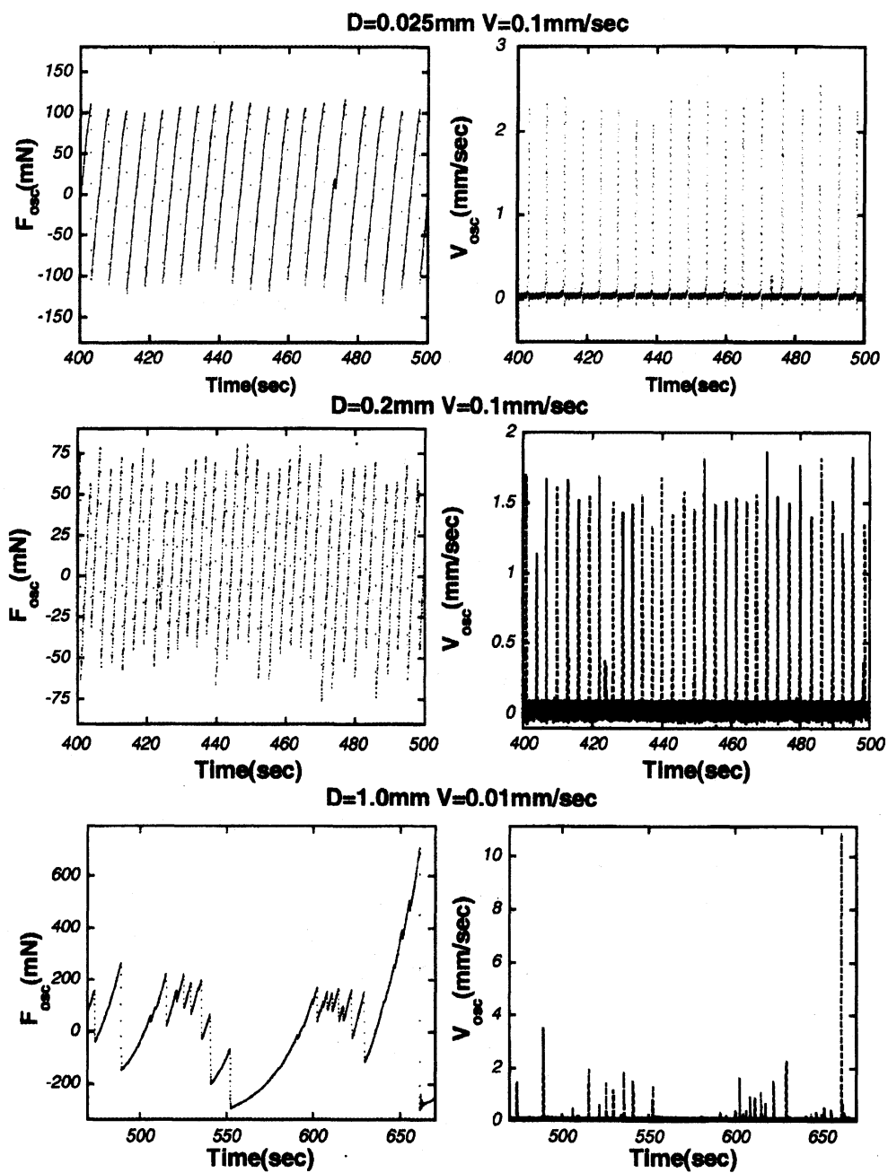
図 5: Stick-Slip の遷移
