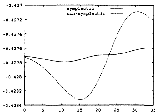
図 4: 蜃気楼が発生している状況で光線追跡を行った場合のエネルギー値
