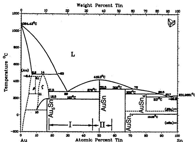
図2 Au-Sn系相図
