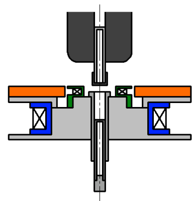
図2 回転角速度の制御部の模式図
