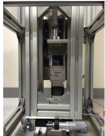
図6 スライド機構の磁石間距離制御部
