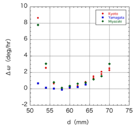
図 4 磁石間距離と角速度の関係
