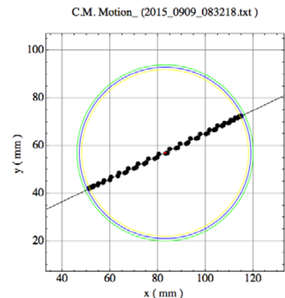
図 3 振子の重心軌道の上面図
