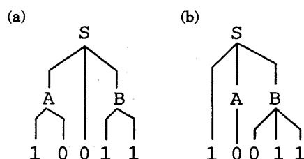
図 1: 解析木の例
