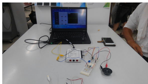
図 1: PC と myDAQ による回路実験の例
