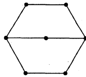
図 1. \theta(1, 2, 2)
