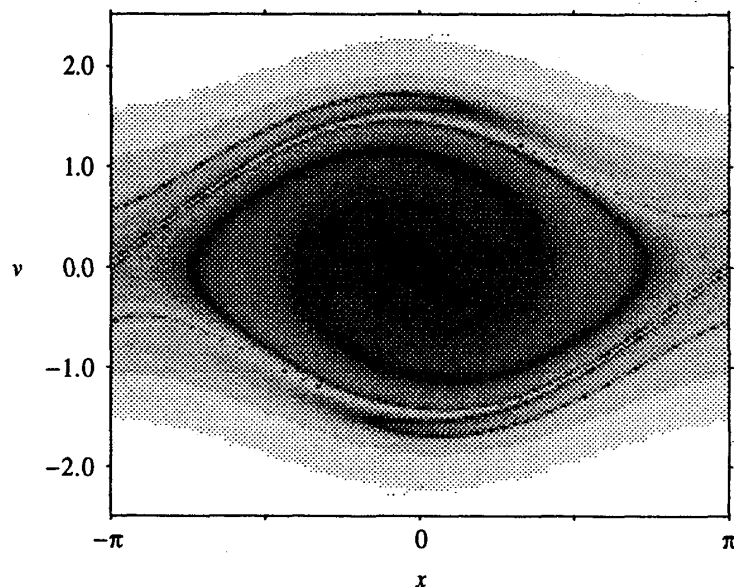
図 1. 1 次元 Jeans 不安定によって発達した、分布関数のフィラメント構造.
