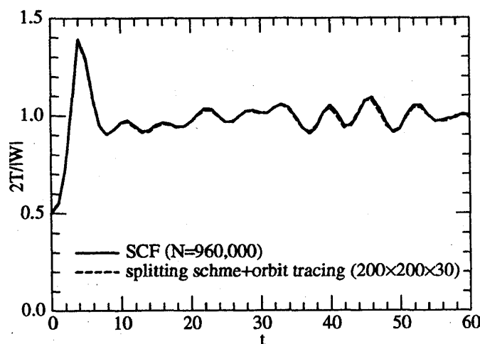
図2. 2つの異なる方法による、一様密度球 (初期のビリアル比 0.5) の collapse でのビリアル比の時間変化.
