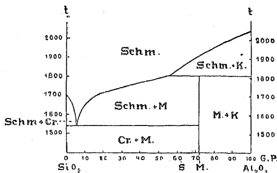
Kristallisationsdiagramm des Systems \text{SiO}_2 - \text{Al}_2\text{O}_3 nach den Angaben von Bowen und Greig.
