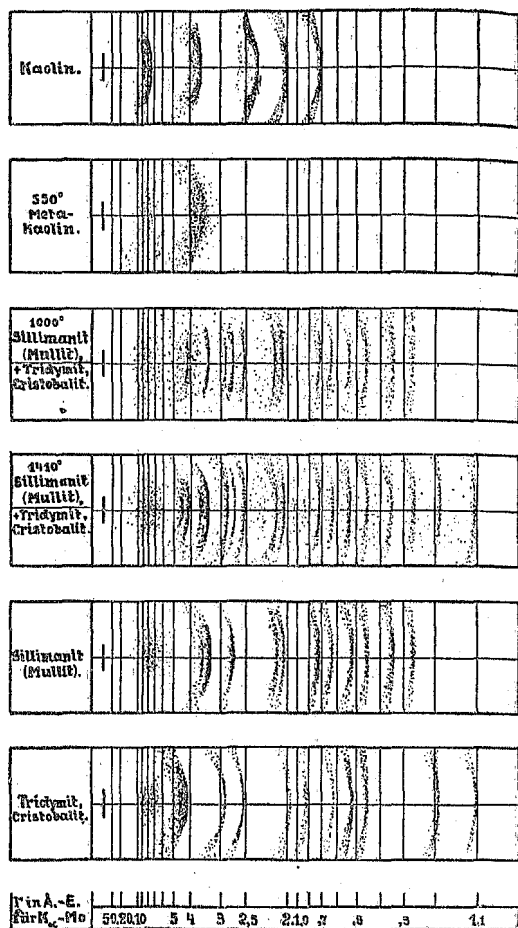
Schemata der Schaukeldiagramme von Kaolin und seiner Brennprodukte.
