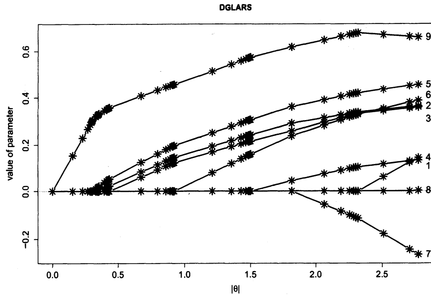
図3 SAHDデータのロジスティック回帰に対するDGLARSの結果。横軸は推定値の l_1 -ノルムを、縦軸はパラメータ \theta^i の値を示している。図の左端からスタートし、右端に到る。
