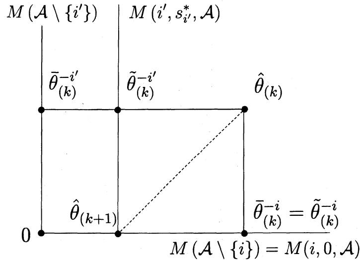
図 1 推定量の更新. \mathcal{A} \subseteq \{1, 2, \dots, d\} : 説明変数を指定するインデックス. M(i, s, \mathcal{A}) = \{\theta \mid \theta^i = s, \theta^j = 0 (j \notin \mathcal{A})\} . 0: 原点. \hat{\theta}_{(k)} : k 番目の推定量. \hat{\theta}_{(k+1)} : k+1 番目の推定量. \bar{\theta}_{(k)}^{-i} : サブモデル M(\mathcal{A} \setminus \{i\}) = M(i, 0, \mathcal{A}) における最尤推定量, あるいは \hat{\theta}_{(k)} の M(\mathcal{A} \setminus \{i\}) への -1 -射影でも同じ. D(\hat{\theta}_{(k)} \mid \bar{\theta}_{(k)}^{-i'}) > D(\hat{\theta}_{(k)} \mid \bar{\theta}_{(k)}^{-i*}) である. \tilde{\theta}_{(k)}^{-i'} : \hat{\theta}_{(k)} の M(i', s_{i'}^*, \mathcal{A}) への -1 -射影. s_{i'}^* : 条件 D(\hat{\theta}_{(k)} \mid \tilde{\theta}_{(k)}^{-i'}) = D(\hat{\theta}_{(k)} \mid \bar{\theta}_{(k)}^{-i*}) より決まる値. \hat{\theta}_{(k)} は M(\mathcal{A} \setminus \{i'\}) よりも M(\mathcal{A} \setminus \{i^*\}) に近いので \tilde{\theta}_{(k)}^{-i*} = \bar{\theta}_{(k)}^{-i*} である. \hat{\theta}_{(k+1)} は M(i^*, 0, \mathcal{A}) と M(i', s_{i'}^*, \mathcal{A}) の交点として定義される. 点線は角の二等分線に対応する曲線である. BR アルゴリズムでは, 推定量がこの曲線に沿って動いていると見ることができる.
