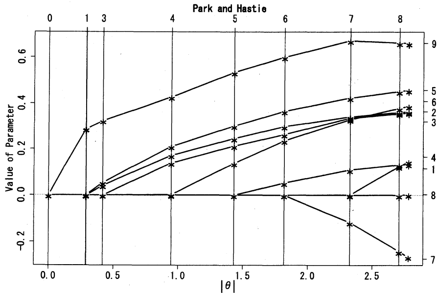
図 4 SAHD データに対する Park and Hastie の方法の結果. 横軸は推定値の l_1 -ノルムを, 縦軸はパラメータ \theta^i の値を示している. 縦線の上の数字は非零成分の個数を示している. 図の右端から左端に見ていくと, パラメータが 0 になる順番は \theta^8, \theta^4, \theta^7, \theta^1, \theta^6, \theta^3, \theta^2, \theta^5, \theta^9 であった.
