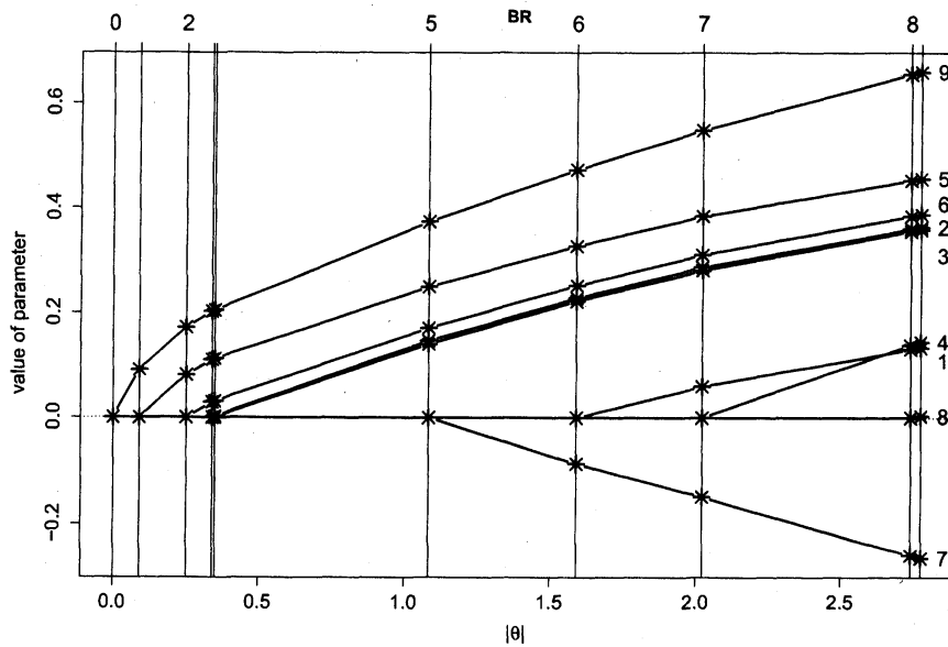
図2 SAHDデータのロジスティック回帰に対するBRの結果。横軸は各推定値の l_1 -ノルムを示している。縦軸は説明変数 x_i ( i = 1, 2, \dots, 9 )の回帰係数 \theta^i ( i = 1, 2, \dots, 9 )の値を表す。図の右端はフルモデルの最尤推定値であり、BRアルゴリズムの出発点を表している。左端はBRアルゴリズムの出力した最後の推定値であり、推定したいパラメータがすべて0になっている。図に入っている縦線はそれぞれBRアルゴリズムが出力した推定値に対応している。左に進むにしたがって非零成分の個数がひとつずつ減っていく。縦線の上の数字は非零成分の個数を示している。パラメータが0になる順番は \theta^8, \theta^4, \theta^1, \theta^7, \theta^3, \theta^2, \theta^6, \theta^5, \theta^9 であった。
