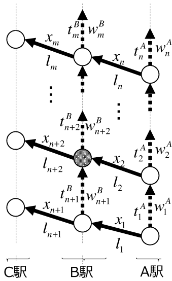
図 25: 接続関係
