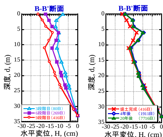
図-17 経過時間に伴う水平変位量 (盛土のり先部)
