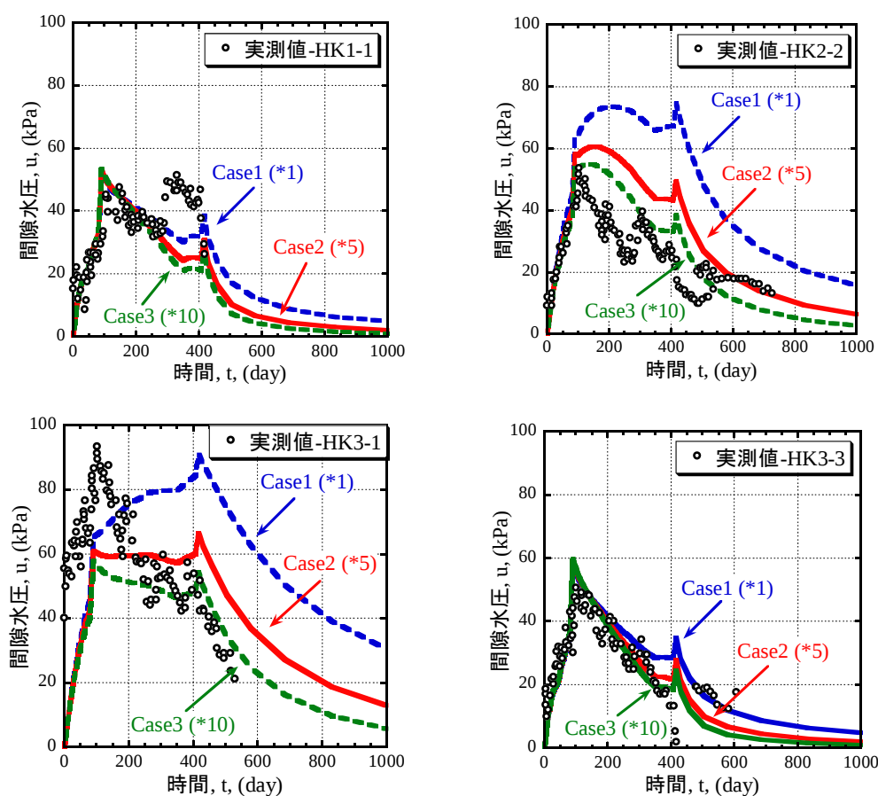
図-20 時間-間隙水圧関係
