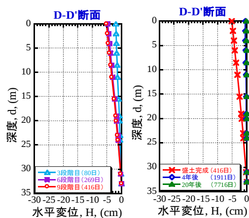
図-18 経過時間に伴う水平変位量 (D-D'地点)
