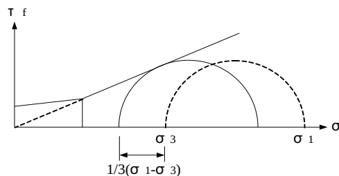
図-7 「有効な全応力」による整理法
