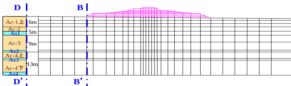
図-16 水平変位対象箇所（Case2）
