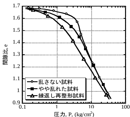
図-6 正規圧密粘土の圧縮曲線
