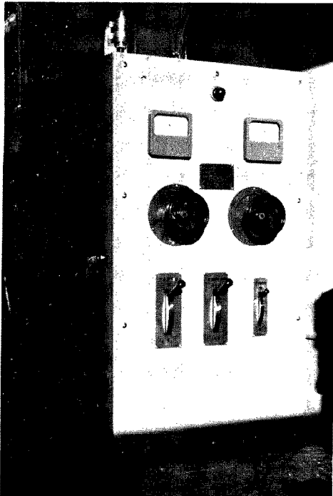
Fig. 25 Silicon rectifier
