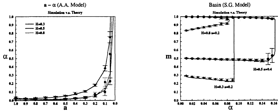
図 1: 左：自己想起モデルの記憶容量とスパースの度合いの関係。実線は理論曲線、エラーバー付データはシミュレーション。右：相互想起モデルでの引き込み領域。実線が理論曲線で下のラインが想起可能な最小初期オーバーラップ、上のラインが想起成功後の最終オーバーラップ。エラーバー付データはシミュレーション。
