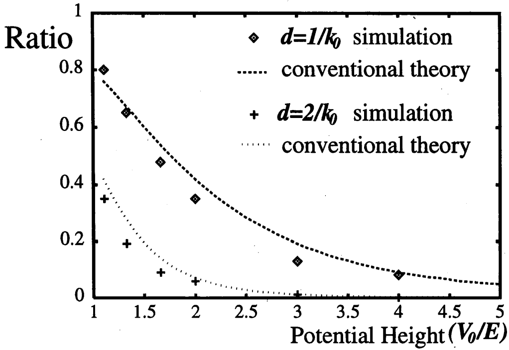
FIG. 3. サンプル数の比と波動関数から計算した反射確率
