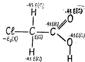
第 1 圖 * \text{Cl}\cdot\text{CH}_2\cdot\text{COOH} 分子内に於ける電荷分布 \epsilon(C_1) = \epsilon_s(\text{Cl}) / (1 + 4 \times .45 + .45^2) \epsilon(O) = .45^2 \epsilon(C_1)
