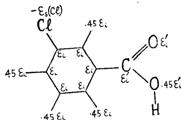
第2圖 m-Cl·C 6 H 4 ·COOH 分子内に於ける誘導電荷の分布 \epsilon_i = \epsilon_s(\text{X}) / (6 + 5 \times .45) \epsilon'_i = .45 \epsilon_i / (2 + .45) \epsilon_m(\text{O}) = .45 \epsilon'_i
