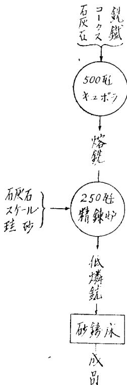
第 2 圖 中間工業實驗操業系統圖
