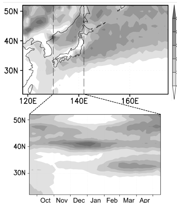
図1 (上) 120–160°E における気候平均の低気圧中心存在頻度(*0.01%/6hr). (下) 130°–140°E で東西平均した低気圧中心存在頻度．
