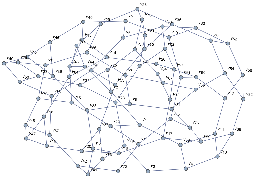
FIGURE 2. G_1(1009, 2) のグラフ
