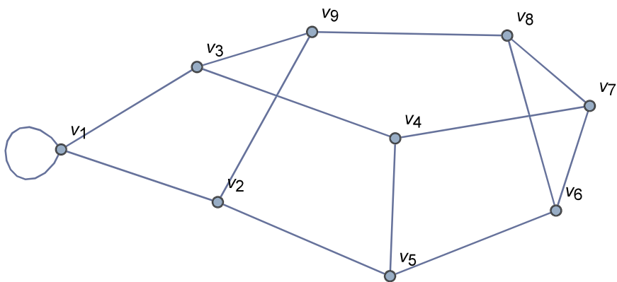
FIGURE 1. G_1(109, 2) のグラフ
