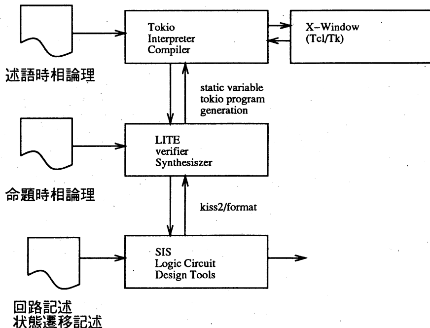
Figure 2: 時相論理プログラム合成システム
