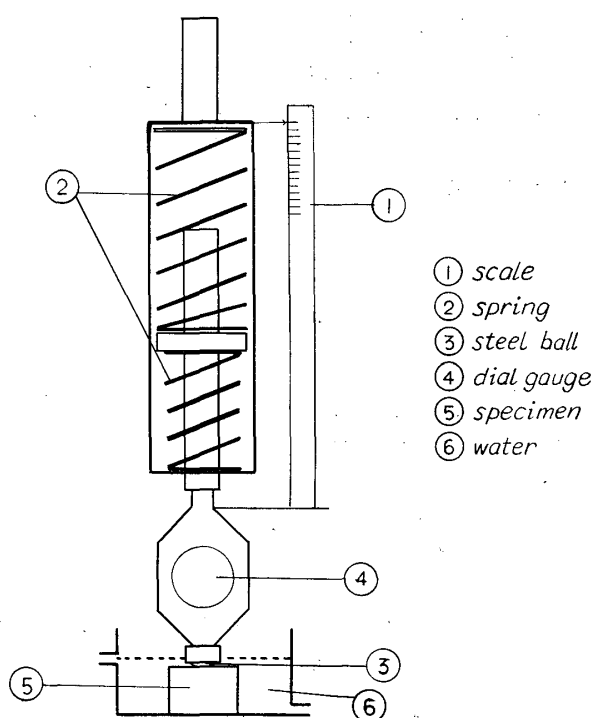
Fig. 1. Apparatus.
