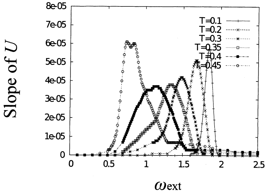
図 2 エネルギー取得率を振動外場の振動数 \omega_{\text{ext}} の関数としてグラフに表した. 相空間 (q, p) の刻みは 128 \times 256 である. エネルギー取得率は内部エネルギー U(t) の 0 \leq t \leq 100 での傾きから得られている.
