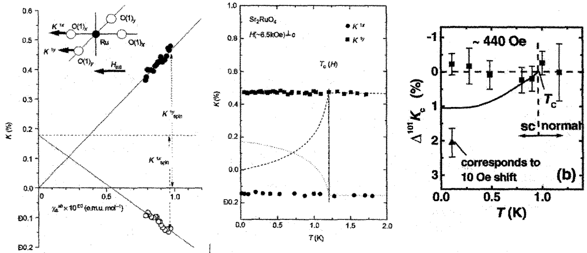
図9: H \perp c と H \parallel c に対する \text{Sr}_2\text{RuO}_4 の Knight shift の温度依存性 [13, 14]
