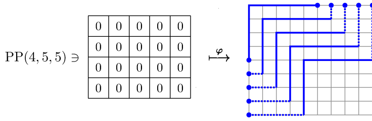
図 6 空の平面分割 \emptyset とそれに対応する非交叉格子路.
