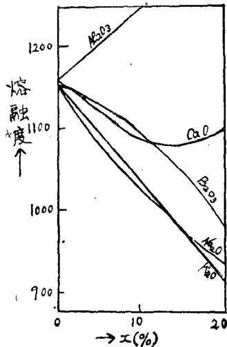
第1圖 \text{Na}_2\text{O} 18% \text{SiO}_2 (82-x)% \text{SiO}_2 の置換による熔融度の 変化 (Gehlhoff 其他の測定値より)
