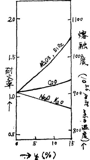
第3圖 基礎釉中の 硼酸置換 \text{SiO}_2 55% \text{Al}_2\text{O}_3 5% \text{CaO} 5% \text{Na}_2\text{O} 15% \text{K}_2\text{O} 5% \text{B}_2\text{O}_3 (15-y)%
