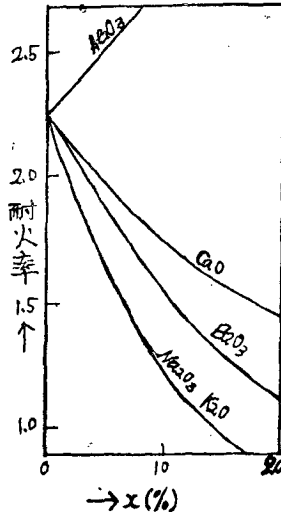
第2圖 \text{Na}_2\text{O} 18% \text{SiO}_2 (82-x)% \text{SiO}_2 の置換による耐火率の 変化 (計算値)
