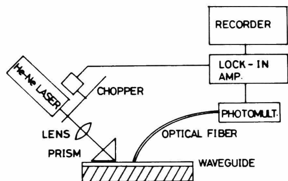
Fig. 7.5 減衰測定装置
