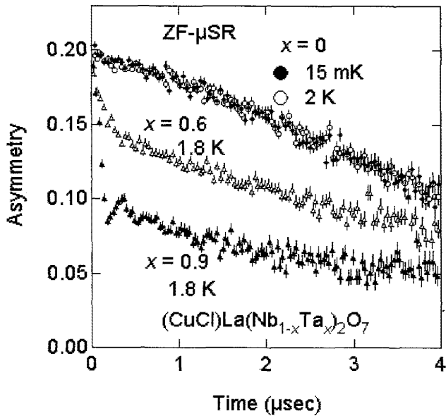
図 4-10 x = 0, 0.6, 0.9 の ZF- \mu SR 測定の結果。 x = 0 について 2 K 及び 15 mK でのスペクトルは基底スピン一重項状態を反映しともに遅い緩和を示した。対して x = 0.9 では t = 0 から速い緩和を示し、基底状態は磁気秩序状態である。これらに対して x = 0.6 では、0.2 \mu sec 程度までの速い緩和と、それ以降の遅い緩和の二種類の成分が観測された。
