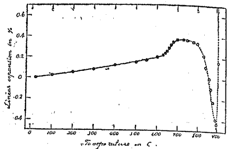
有田産黒曜石の加熱による膨脹線
