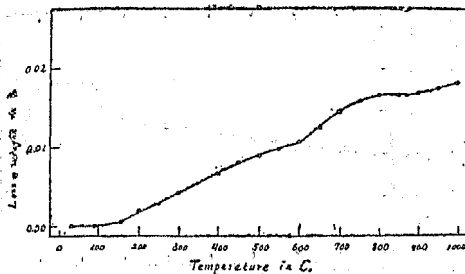
豊後國姫産流紋岩玻璃の加熱による重量變化
