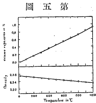
容るす對に度溫の石曜黑産田有 (照參表三第) 化變の重比及積
