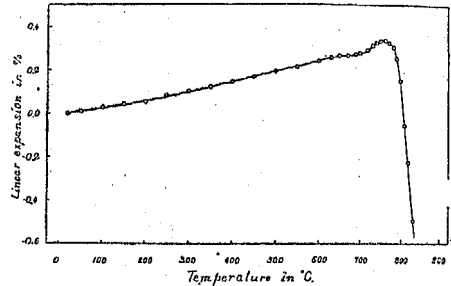
三宅島のリピラ熔體の加熱による膨脹線
