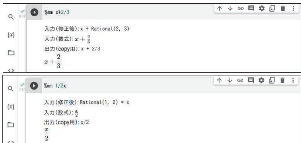
図 10: 簡易文法修正マジックコマンドの実行例（分数の取り扱い）
