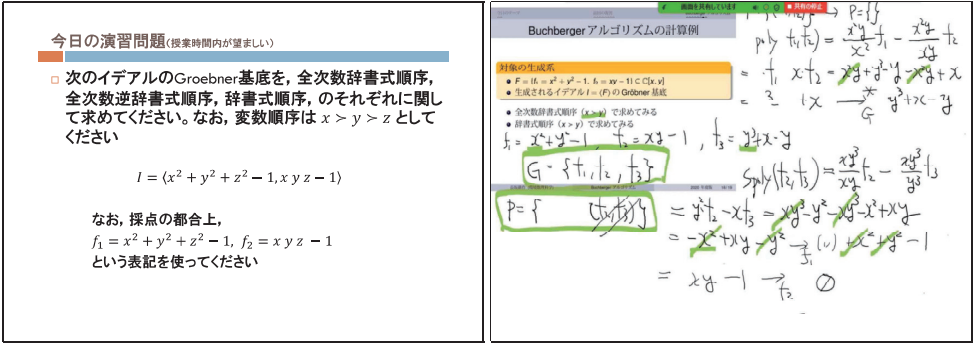
図 1: Gröbner 基底を計算する Buchberger アルゴリズムに関する授業資料
