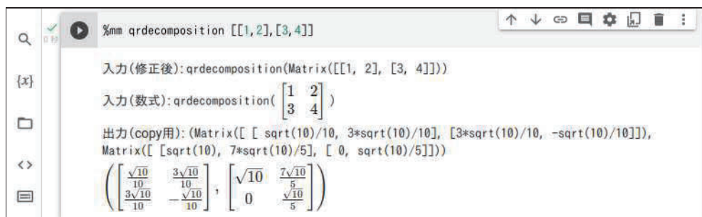
図 9: 簡易文法修正マジックコマンドの実行例（QR 分解）
