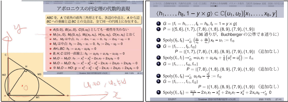
図 2: 有理関数体上で Gröbner 基底を計算する初等幾何の証明に関する授業資料
