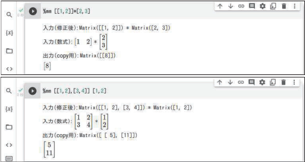
図 7: 簡易文法修正マジックコマンドの実行例（行列の積やベクトルの解釈）
