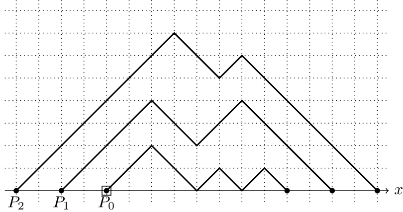
図 2. 非交叉径路 \mathbf{P} = \{P_0, P_1, P_2\} \in \mathbf{P}(4, 3) ( x 軸上の小四角は原点 (0, 0) を指す).
