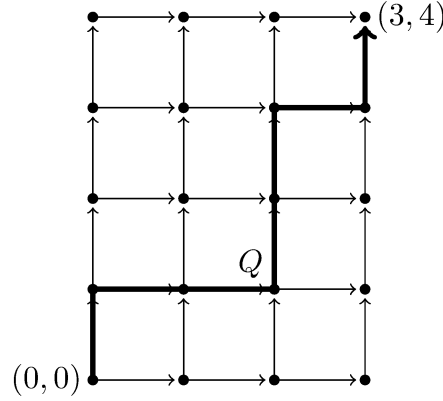
図 5. グラフ G = G(4, 3) と G -径路 Q .
