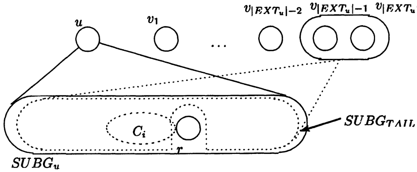
図 3: 補題 5
