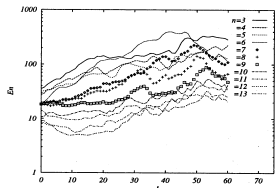
図 4.3.6 モーダルエネルギー (run13)
