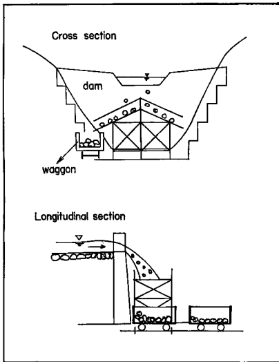
Fig. 8 Sabō-dam type.
