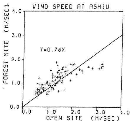
図9-(1) 芦生風速
