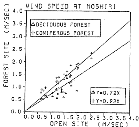
図9-(2) 母子里風速
