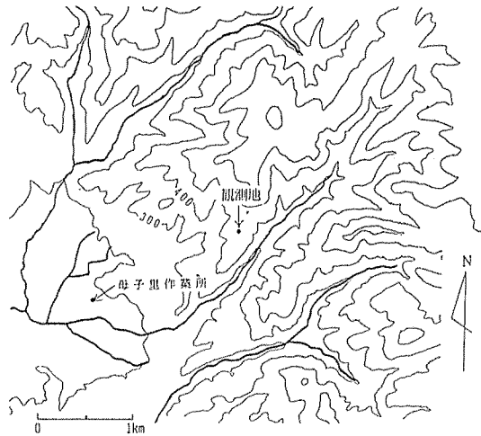
図3 母子里
