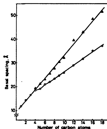
図6. リン酸ジルコニウムアルキルエステル誘導体の層間距離 (O) アルキルアルコール (Δ) アルキルアルコールリン酸塩
