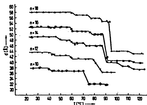
図3. アルキルアンモニウム-粘土-アルコール複合体の層間距離の変化
