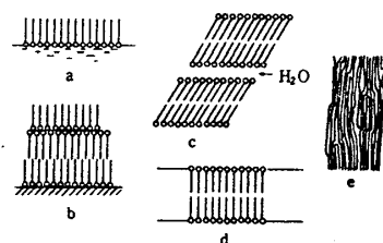
図2. アルキル鎖の配列
