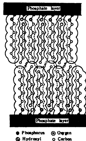
図8. アルコールで誘導した誘導体の構造
