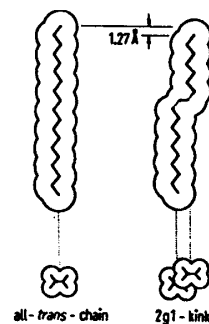
図4. キンクの形成と鎖長の変化
